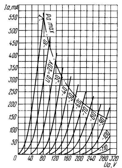
Усредненные анодные характеристики (при работе с одним катодом): U_t = 6,3 В; — — — наибольшая допустимая мощность, рассеиваемая анодом ( P_{a \max} )
