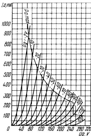
Усредненные анодные характеристики: U_t = 12,6 В; — — — наибольшая допустимая мощность, рассеиваемая анодом ( P_{a \max} )
